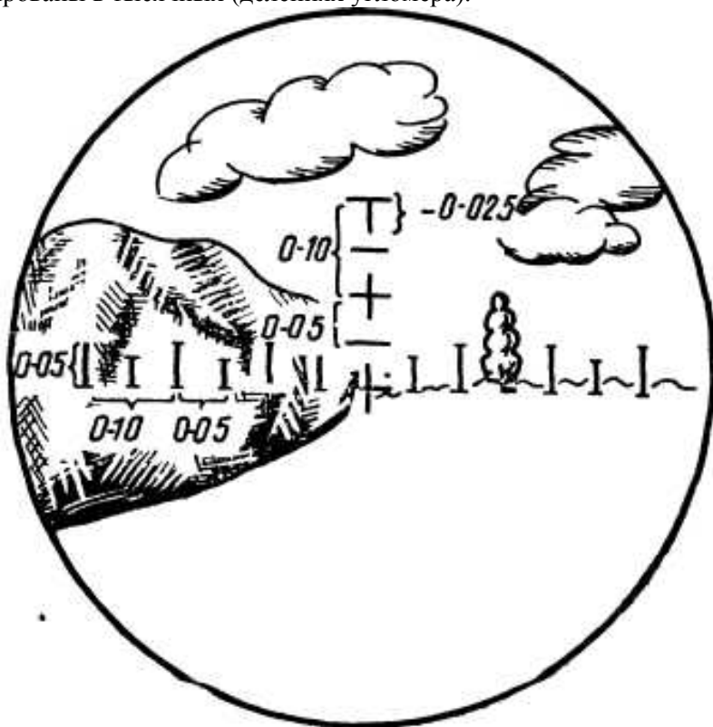
Рис. 71. Углоизмерительная сетка бинокля Б-15
