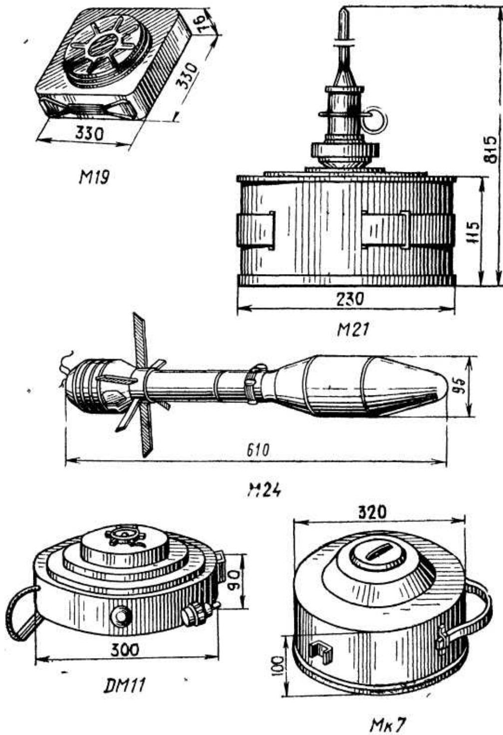
Рис. 144. Противотанковые мины
