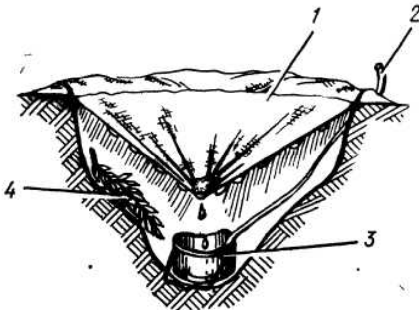
Рис. 87. Устройство солнечного конденсатора:
